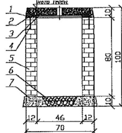
РАЗРЕЗ А-А
