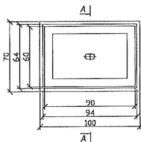
ДЕТАЙЛ - ШАХТА 60/90
